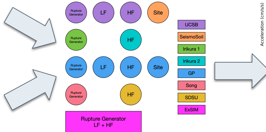
BBP Modules
